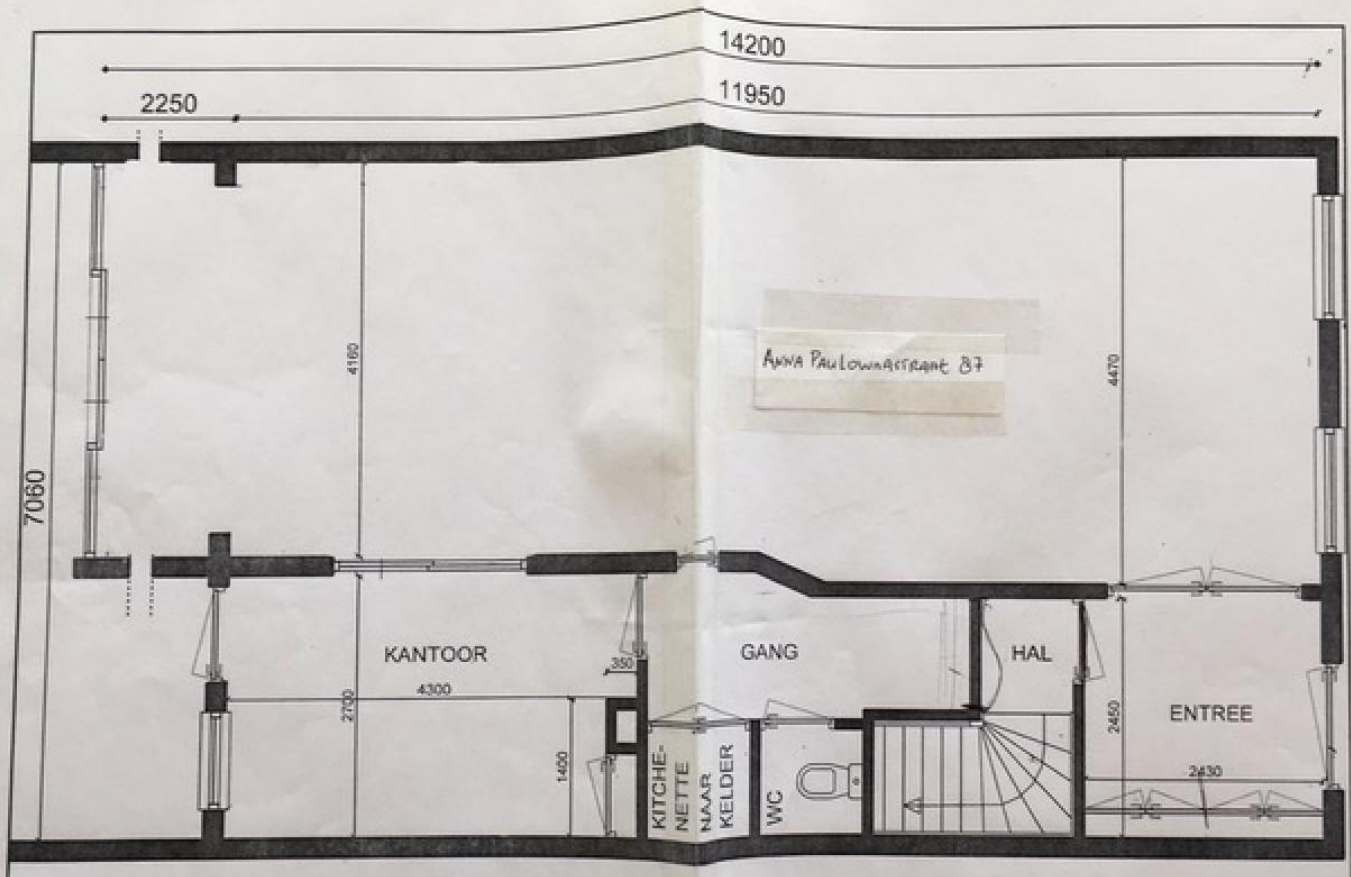
BEGANE GROND - BESTAND
