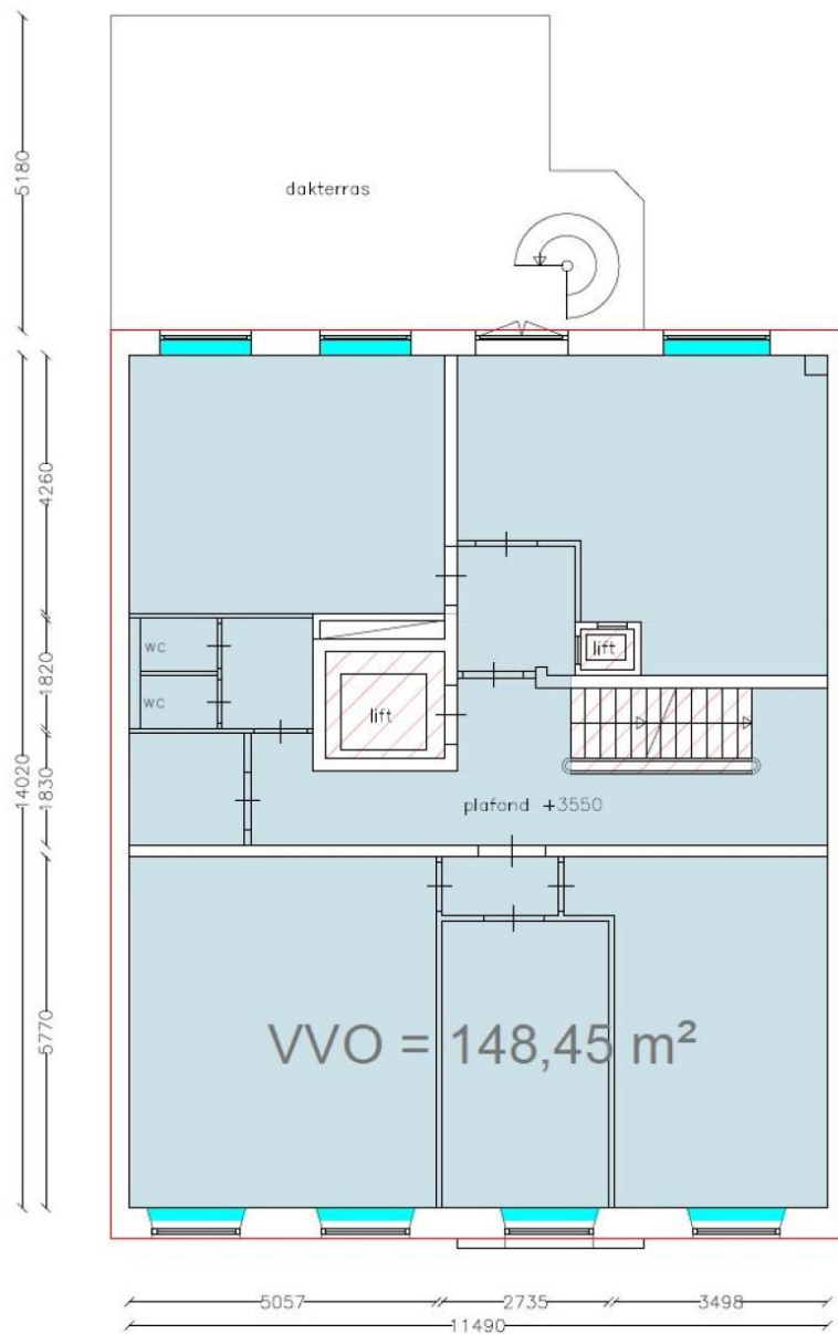
BOUWLAAG 3 - 1e VERDIEPING
