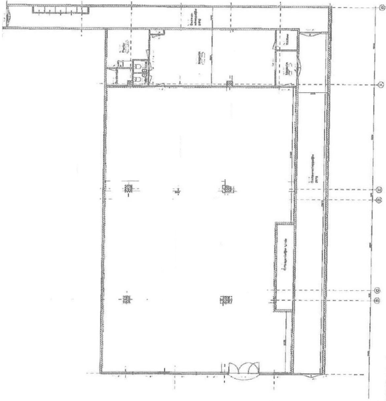
Begane grond
