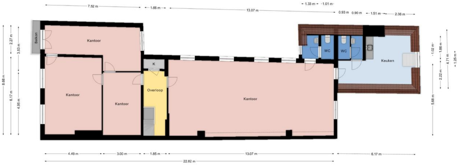
LANGE VOORHOUT 12-12A DEN HAAG 1e Verdieping | h = 3,15 m © m2Vp.nl 2026
