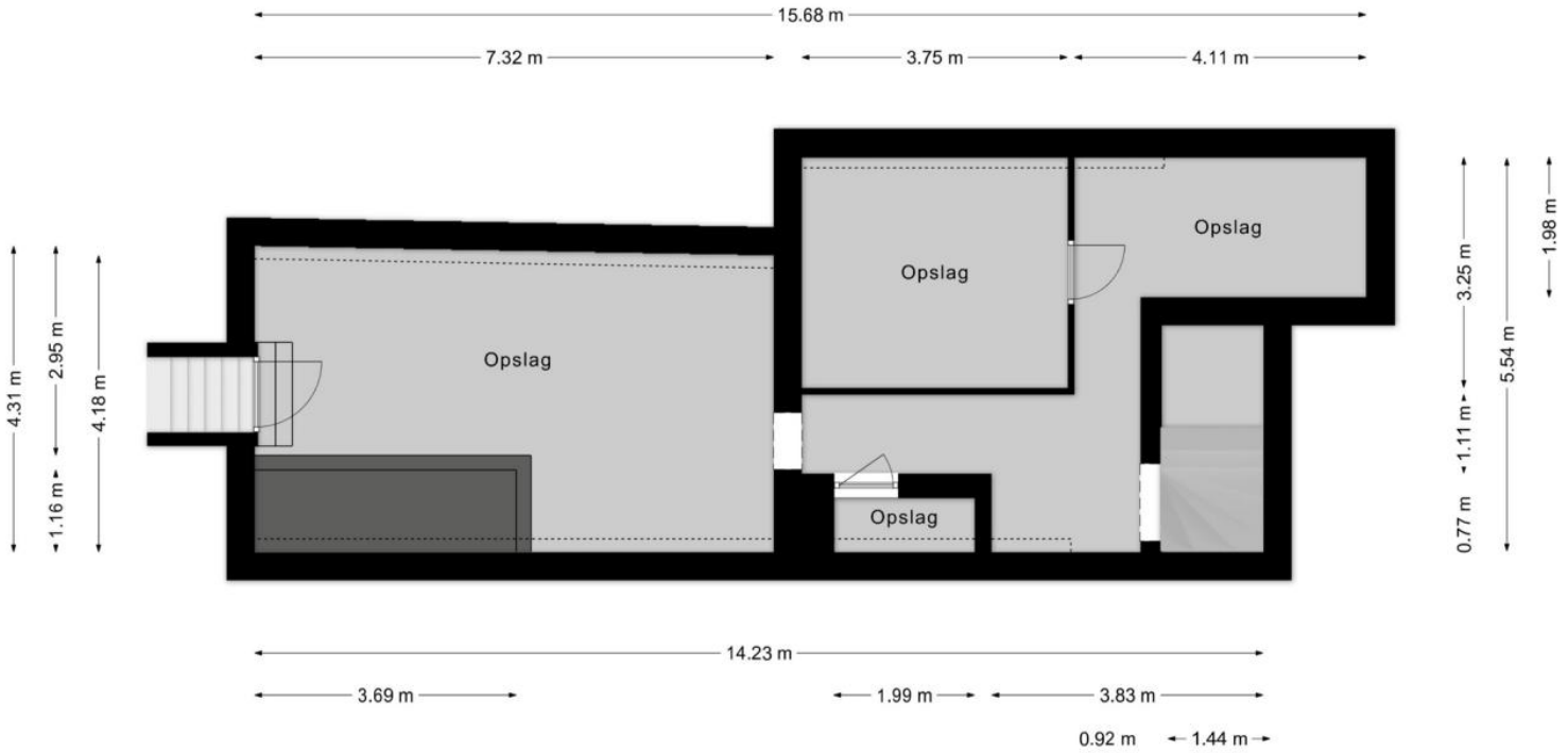
LANGE VOORHOUT 12-12A DEN HAAG Kelder | h = 2,20 m © m2Vp.nl 2026
